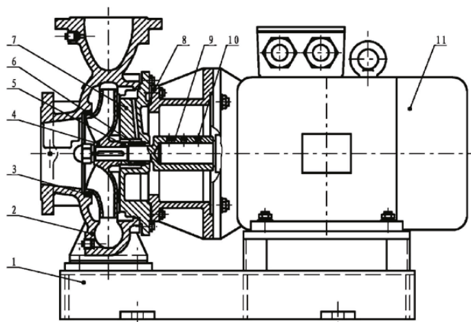
1. Опорное основание 2. Корпус 3. Щелевое уплотнение 4. Рабочее колесо 5. Стопорное кольцо механического уплотнения 6. Механическое уплотнение 7. Корпус уплотнения 8. Фонарь 9. Вал насоса 10. Винты вала 11. Электродвигатель
