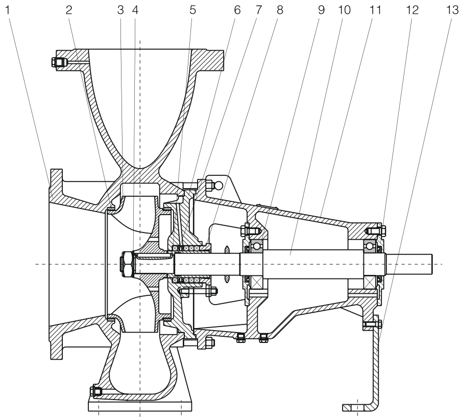
1. Корпус насоса 2. Кольцевое уплотнение 3. Рабочее колесо 4. Гайка рабочего колеса 5. Втулка 6. Задняя крышка насоса 7. Механическое уплотнение 8. Крышка уплотнения 9. Подшипник 10. Вал 11. Фонарь 12. Крышка подшипника 13. Опора фонаря
